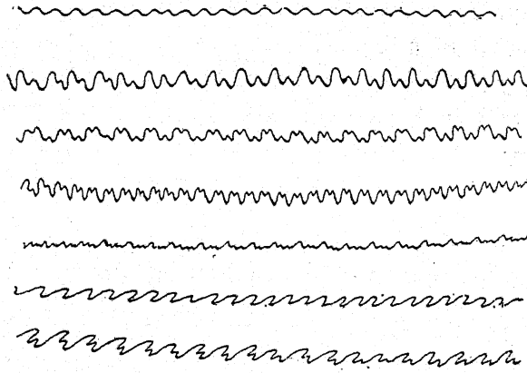
चित्र १४८—लहरों के विविध रूप
